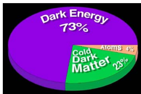
Abbildung 6.1: Anteile der Energie/Massen-Dichte an der Gesamtdichte des Universums, die etwa gleich der kritischen Dichte (siehe (2.16, 2.18)) ist.
