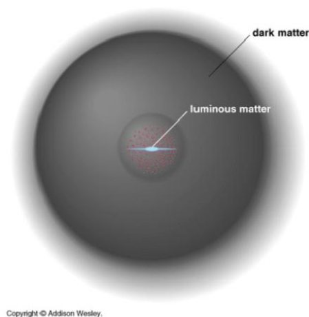
Abbildung 6.3: Schematische Darstellung des DM-Halos um eine Galaxis.
